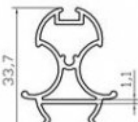
K4402 FİTİLLİ DİKME (KAYAR) (0.420 Kg/m)
