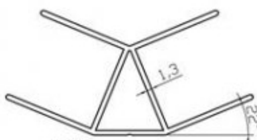
K4410 KOŞE PROFİLİ (135°) (0.570 Kg/m)
